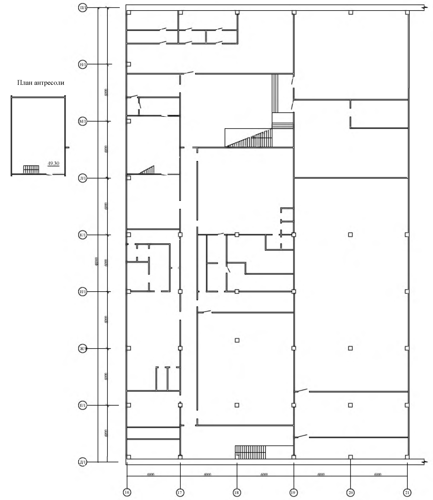
План на отм. + 4.2 м корпуса К-38 А
